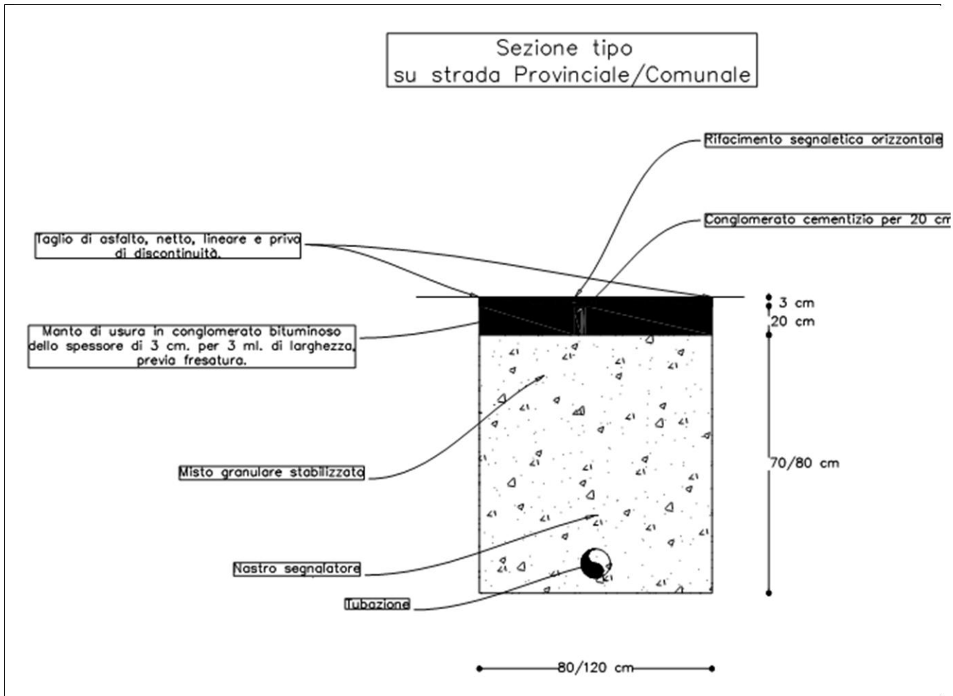
Manutenzione puntuale su tubazione idrica su STRADA PROVINCIALE/COMUNALE
