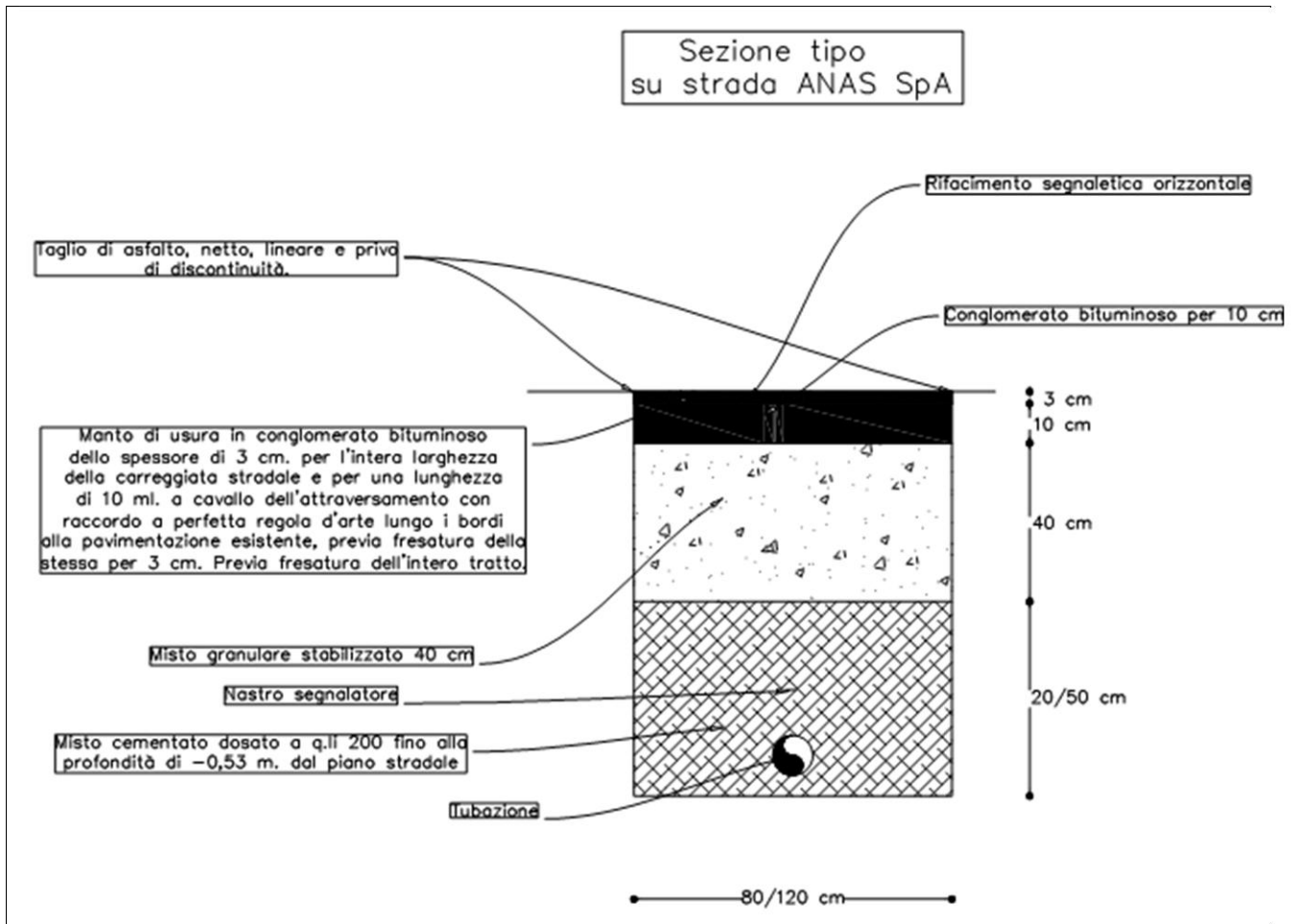
Manutenzione puntuale su tubazione idrica su strada ANAS
