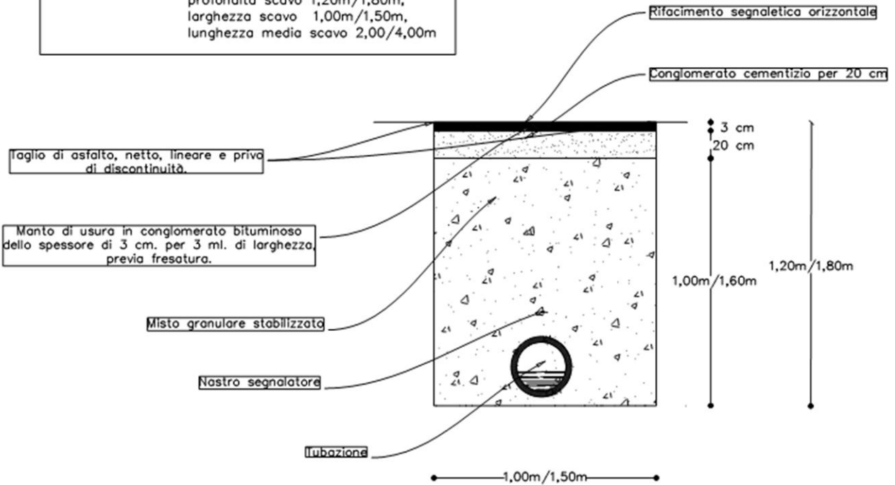
Manutenzione tubazione fognaria su strada Provinciale/Comunale (DN 315/500 mm)
