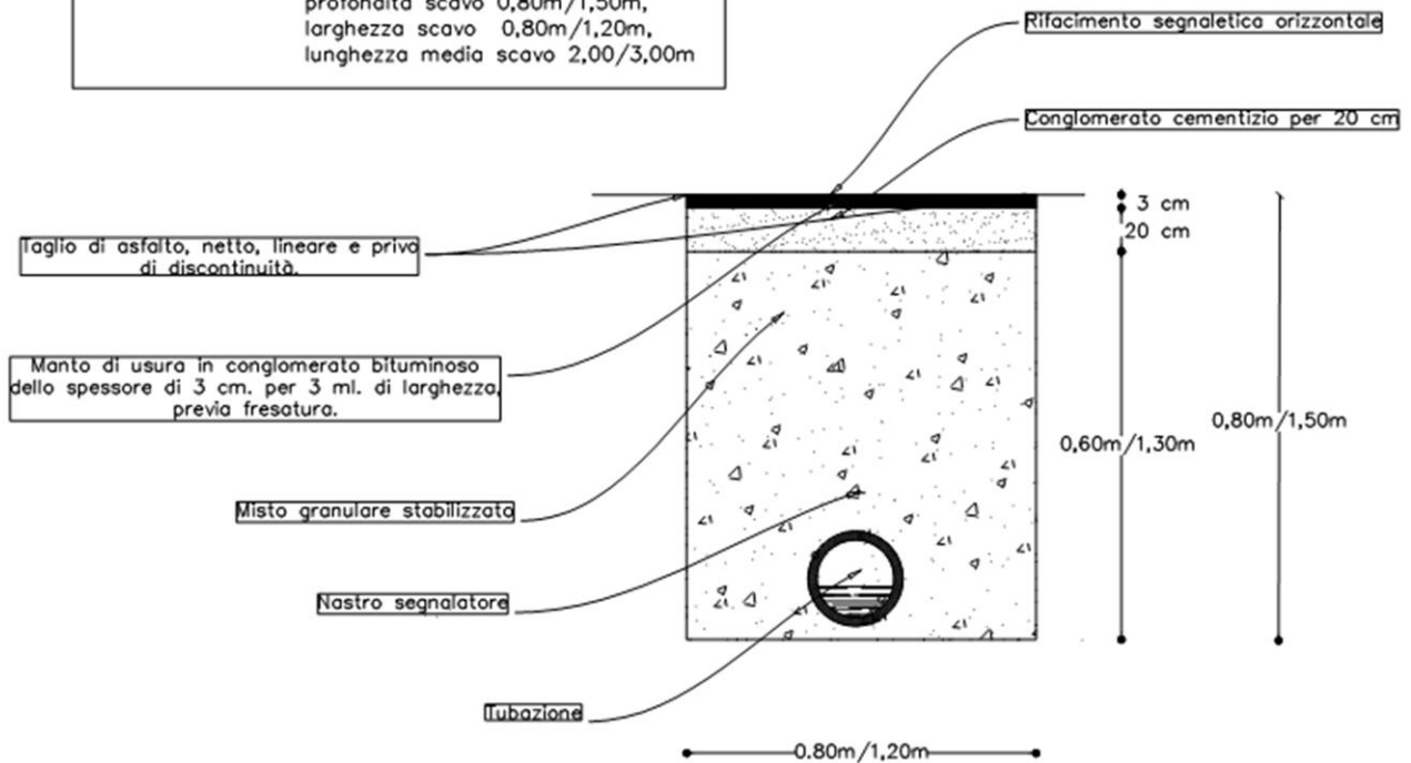
Manutenzione tubazione fognaria su strada Provinciale/Comunale (DN 160/250 mm)
