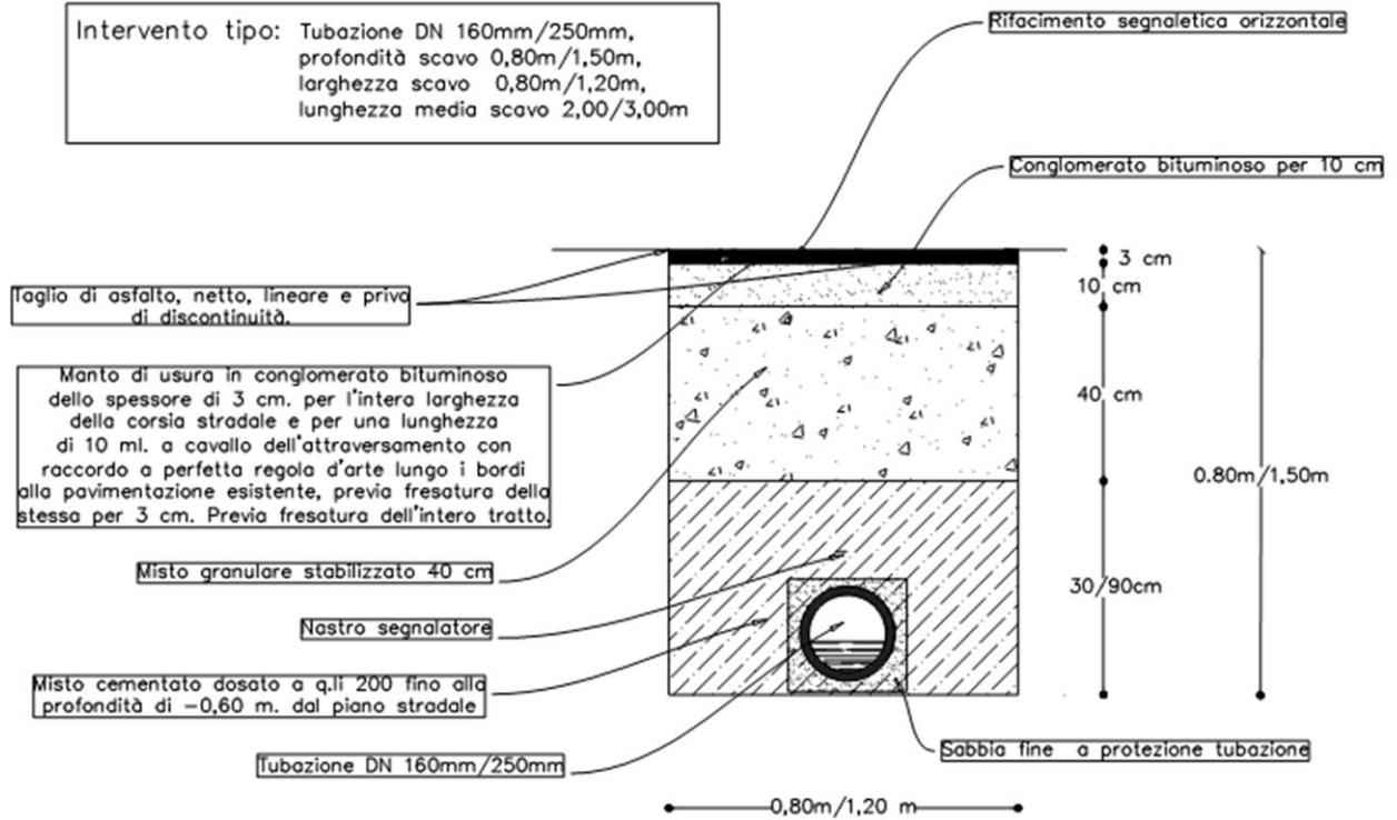
Manutenzione tubazione fognaria su strada ANAS (DN 180/250 mm)
