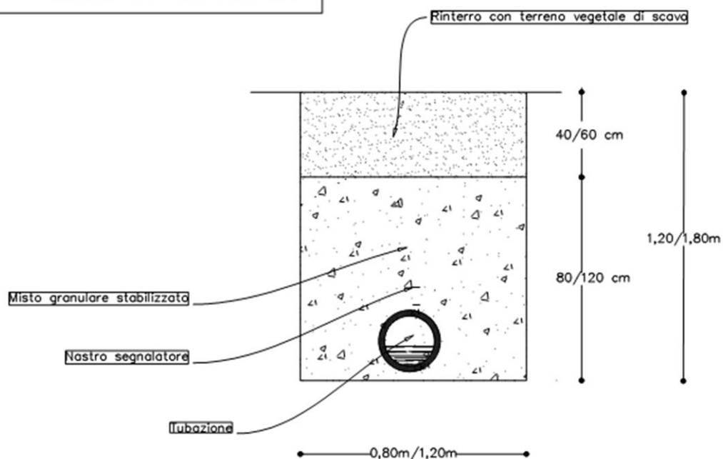
Manutenzione tubazione fognaria su terreno (DN 400/500 mm)
