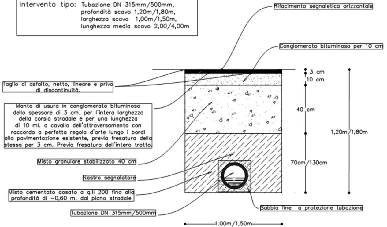
Manutenzione tubazione fognaria su strada ANAS (DN 315/500 mm)
